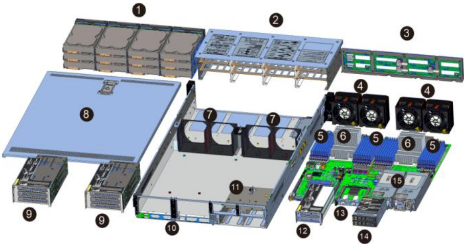
结构图 1-3
