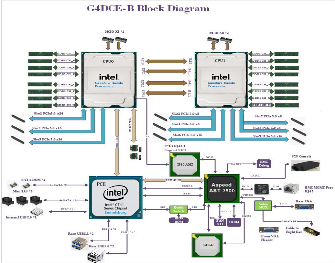
主板逻辑框图 1-2
