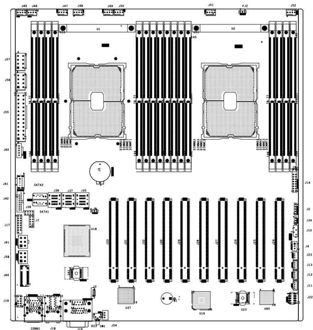
主板图 2-13
